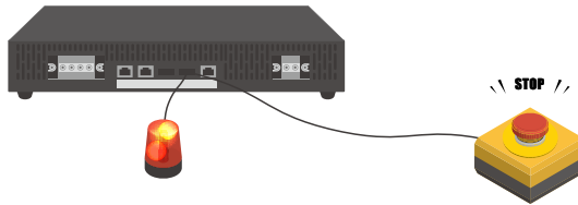
DIO 緊急停止機能使用例
